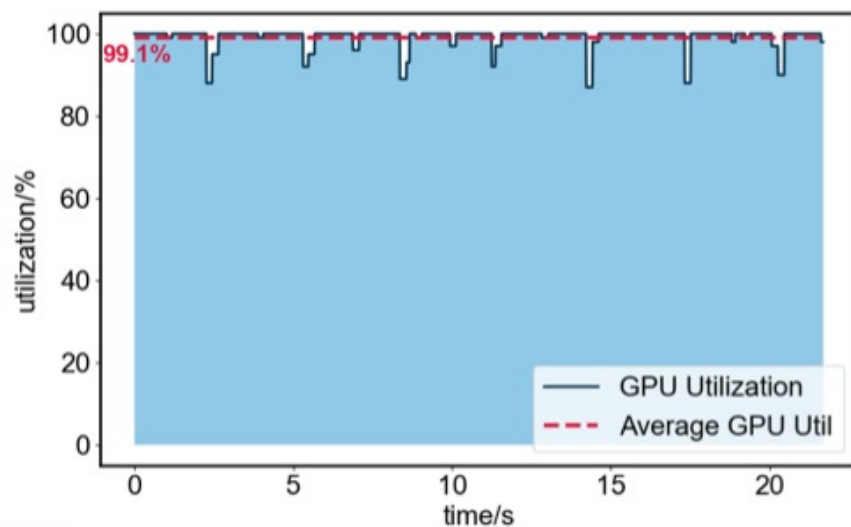
Pytorch
